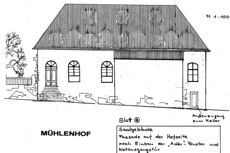
Bild: Neu geplante Fassade des Saales, Hofseite
